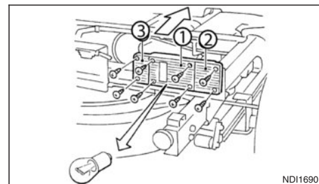
Tylna lampa zespolona (kierunkowskaz, światło hamowania i światło cofania) (modele bez skrzyni ładunkowej)
