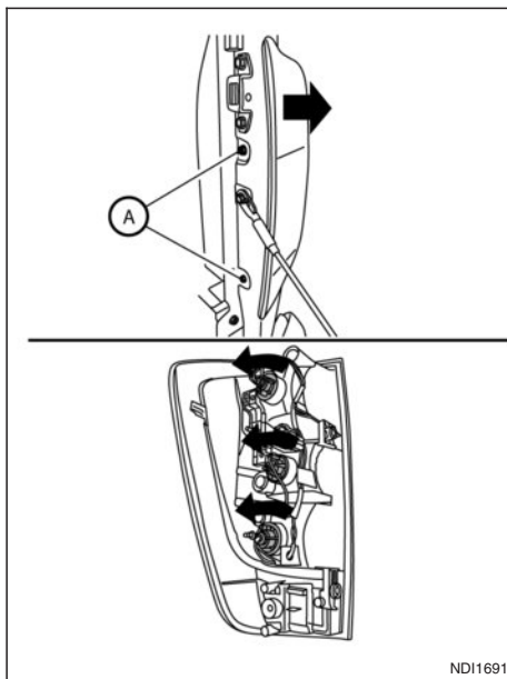
Tylna lampa zespolona (kierunkowskaz, światło hamowania, tylne światło przeciwmgłowe (jeśli na wyposażeniu) i światło cofania) (modele ze skrzynią ładunkową)
