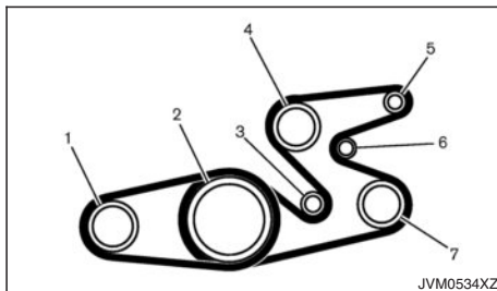
Silnik M9T 2.3DCI
