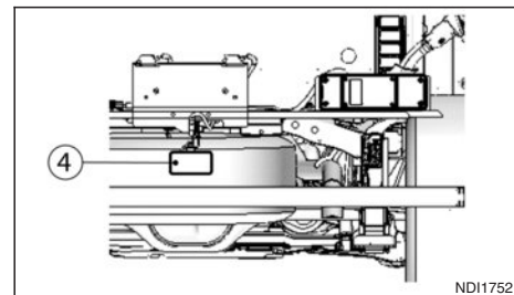
Tylne światło przeciwmgłowe (jeśli na wyposażeniu w pojazdach bez skrzyni ładunkowej)
